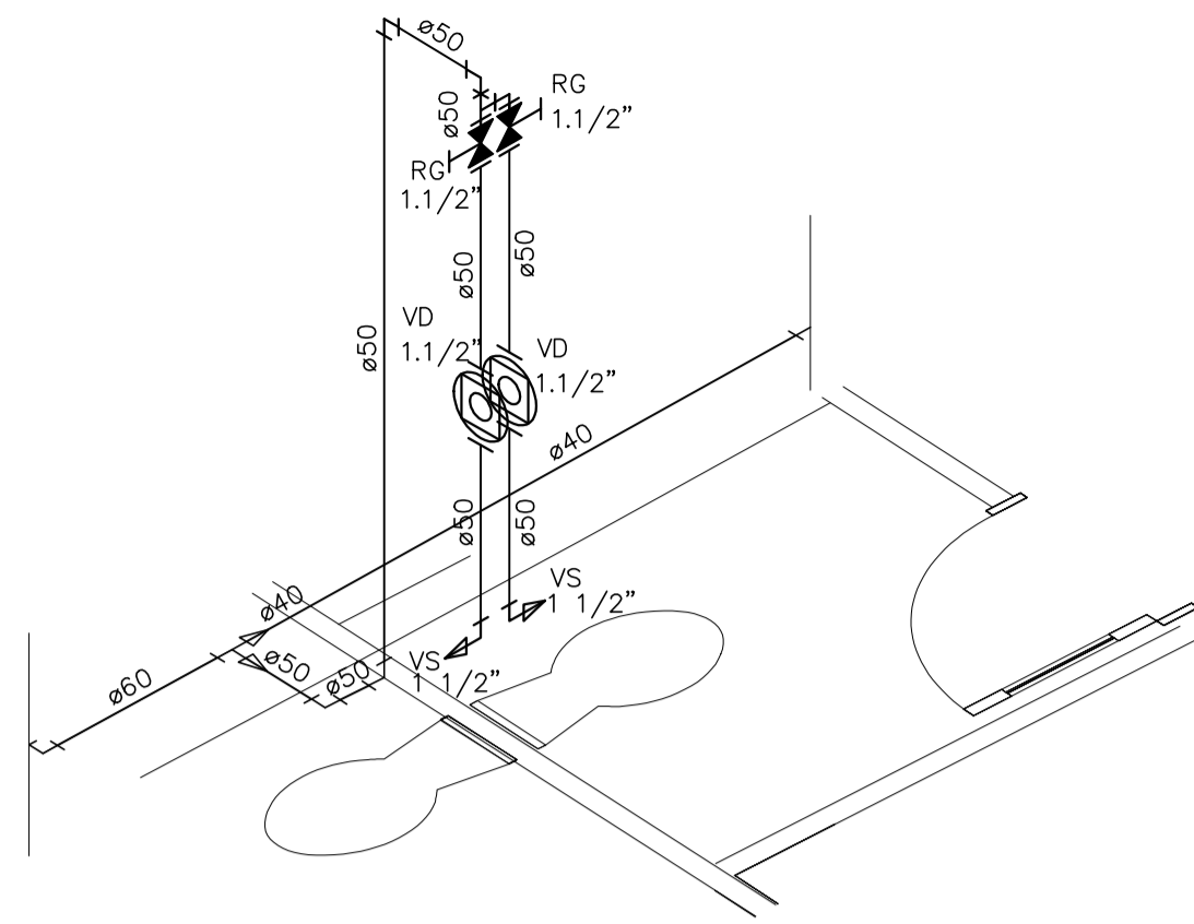
DETALHE H2
